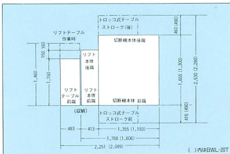
BWL-28T設置スペース テーブル面高さ 820 (820)mm 全 高 2,080 (2,045)mm
